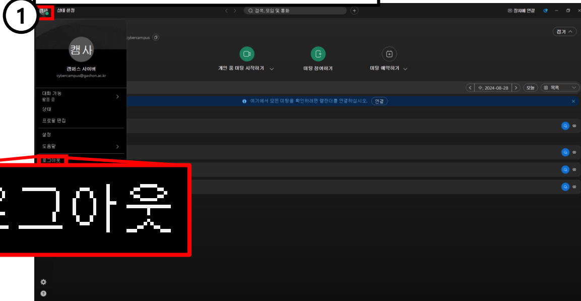
① 「Webex로그아웃」_PC화면
